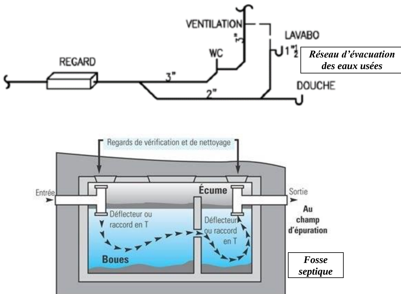
Figure 5 : Schémas relatifs aux installations sanitaires
